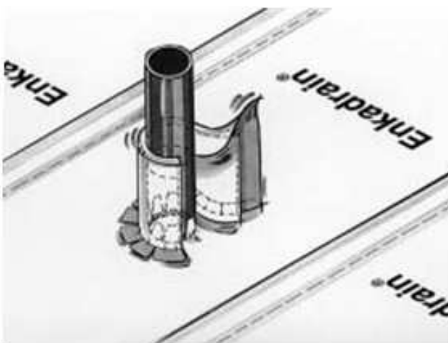
3 Szellőző és ereszcatorna csatlakozás
